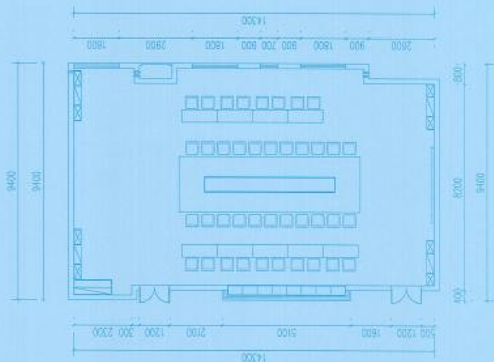
二 平面布置图 SCALE:1:50
